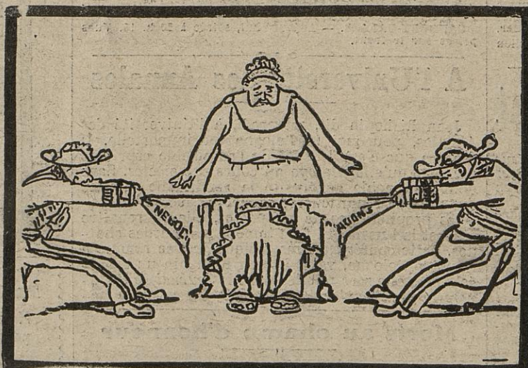
— L'amitié italo-allemande.
