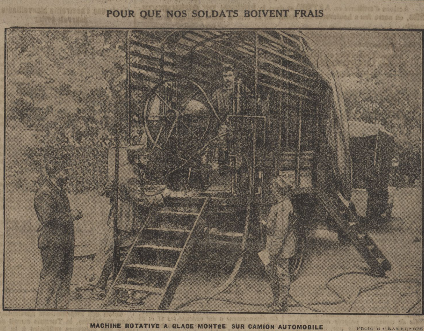
MACHINE ROTATIVE A GLACE MONTÉE SUR CAMION AUTOMOBILE
