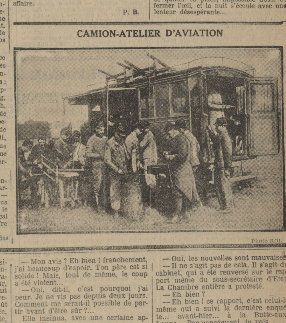
CAMION-ATELIER D'AVIATION. Photo ROU.
