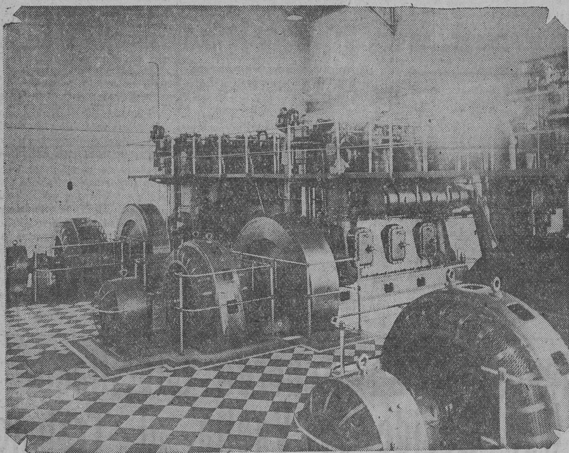
SALA DE MAQUINAS DE LA USINA DE RAFAELA
