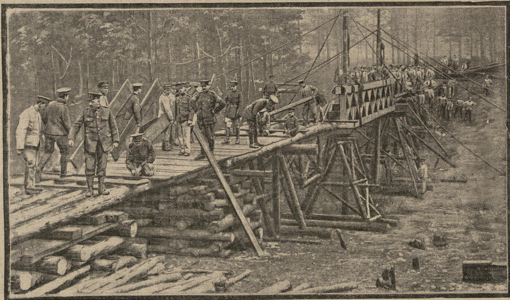
L'instruction des recrues anglaises incorporées dans l'arme du génie se poursuit avec activité. Près du camp d'Aldershot un détachement de ces jeunes soldats construit un pont de bois. Leur entraînement terminé, ces volontaires seront dirigés sur la France, où ils prendront rang dans les armées alliées actuellement sur le front.
