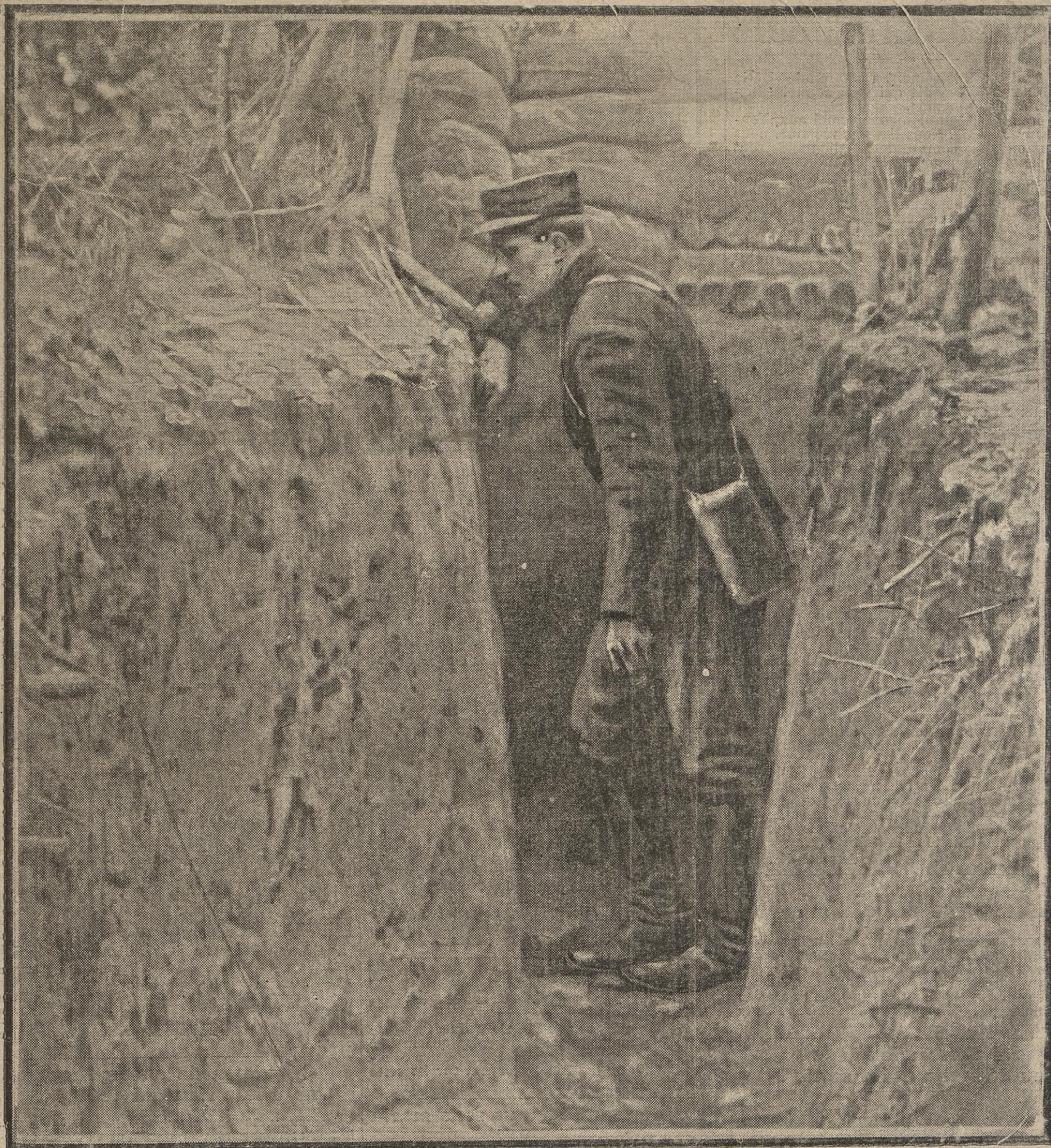
Pour repérer le tir d'une batterie, un sous-lieutenant d'artillerie s'est placé dans une tranchée de première ligne. Afin de communiquer avec son chef de groupe placé à l'arrière et de le renseigner sur l'efficacité du feu de nos 75, l'officier ingénieux, qui ne dispose pas d'un téléphone, se sert d'une vieille gouttière qu'il a transformée en tuyau acoustique.
