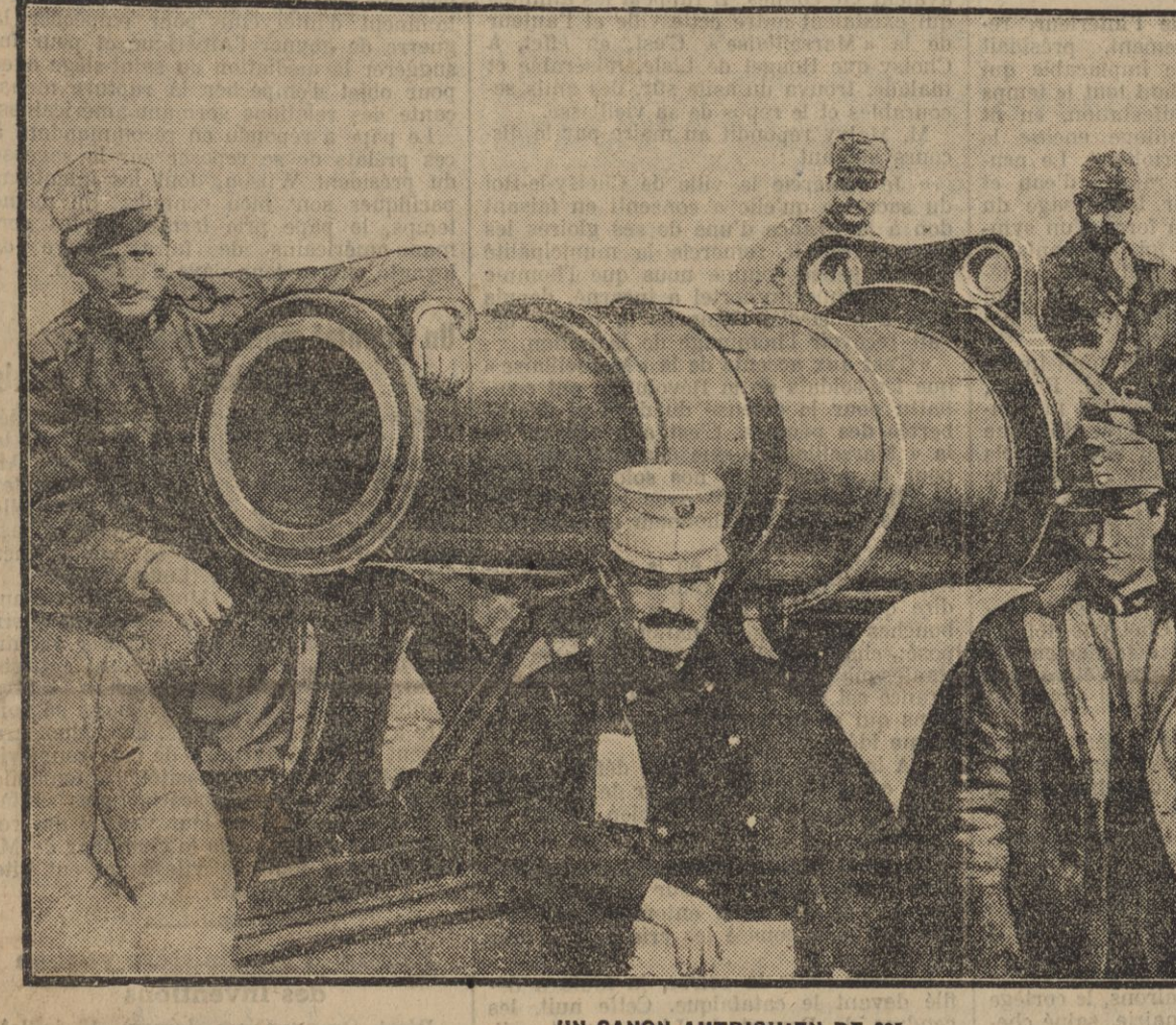
UN CANON AUTRICHIEN DE 305
