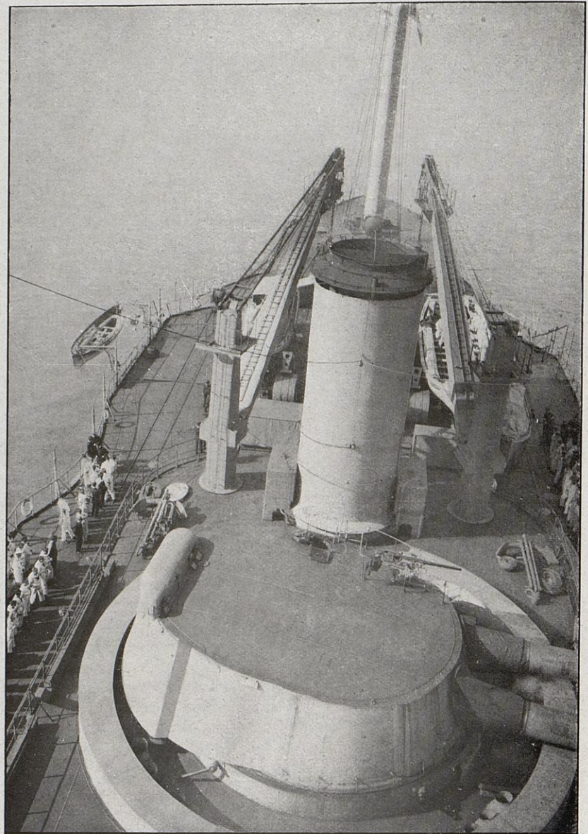
La manœuvre, le ravitaillement, le pointage de ces énormes pièces sont assurés électriquement et automatiquement.
