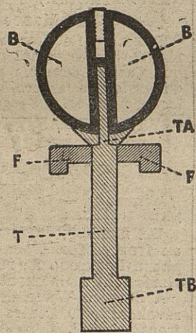
SCHÉMA DU MINENWERFER
