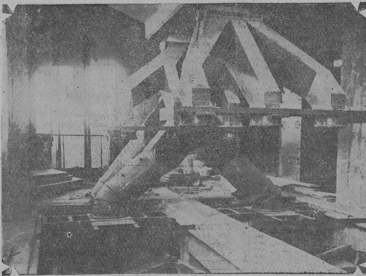
DEPARTAMENTO DE EXPEDICION Y EMBOLSADERO DEL ELEVADOR TERMINAL COOPERATIVO DE ROSARIO
