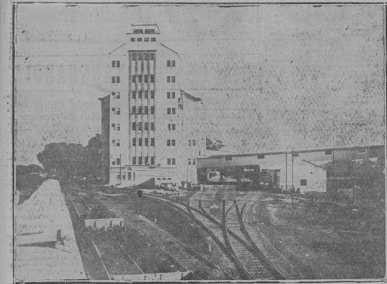
HERMOSO ASPECTO QUE PRESENTA LA PARTE ANTERIOR DEL GRAN ELEVADOR TERMINAL COOPERATIVO que se inaugurará hoy domingo en la ciudad de Rosario. El amplio edificio para maquinarias y oficinas tiene una altura de más de 50 metros y consta de dos subsuelos, además de los nueve pisos que pueden verse en el grabado. Las maquinarias son del tipo más moderno y perfeccionado, característica ésta que, prima hasta en el menor detalle, de esta trascendental obra, que constituye un legítimo motivo de orgullo para el país. En primer plano se ven los desvíos, que en número de tres llegan hasta la casa de recepción, y por los cuales circulan los vagones cargados con el cereal, para ser depositado en los silos. A la derecha, partiendo del primer piso del edificio de maquinarias, está el puente de embarque, del cual la fotografía muestra el comienzo y que tiene un largo de cien metros, terminando en el río.
