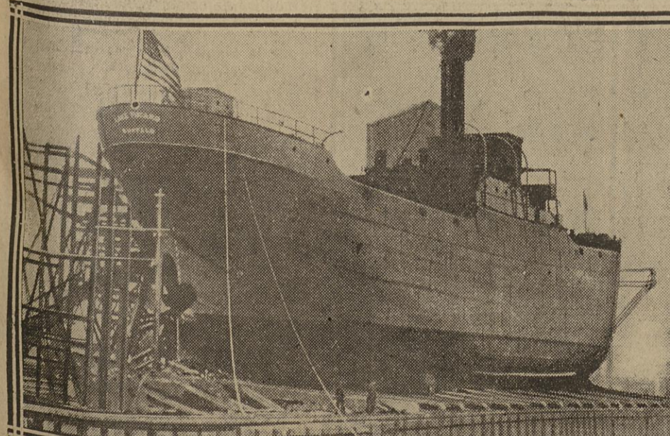
LE NAVIRE GLISSE SUR LA CALE
